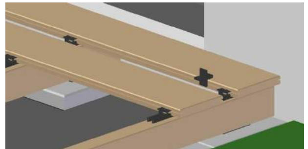
Bild 10. 2 Dielen bis an den Abstandshalter schieben.
