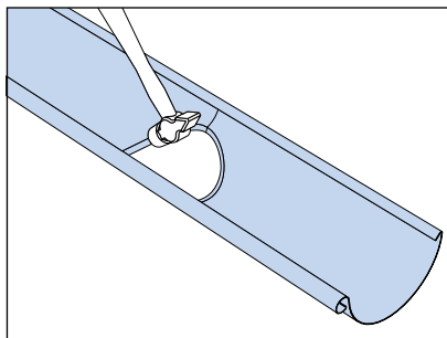
5. Um sicherzustellen, dass das gesamte Regenwasser aus der Regenrinne in den Rinnenablauf gerät, muss die geschnittene Kante mit einem Hammer oder einer Zange etwas nach unten gebogen werden.
