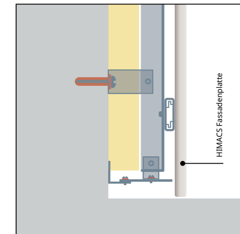
Sockel-Abschluss (unterer Abschluss)
