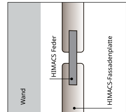
Nut- und Feder-Verbindung (mit Feder-Element aus HIMACS)
