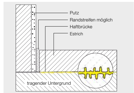
Skizze: Verbundestrich
