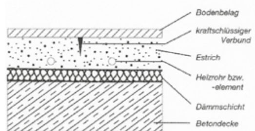
Skizze: Ausführung von Scheinfugen ohne Fuge im Belag
